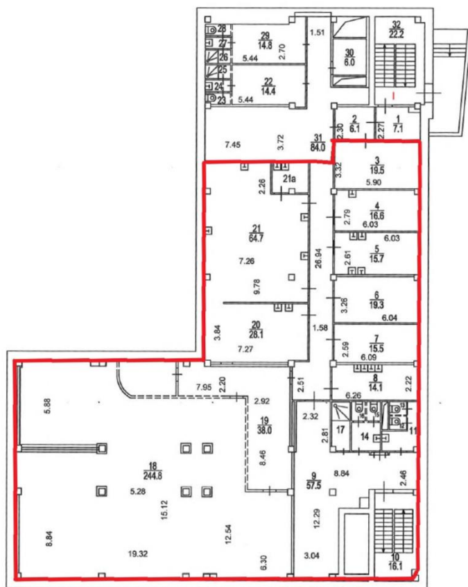
цокольный этаж
